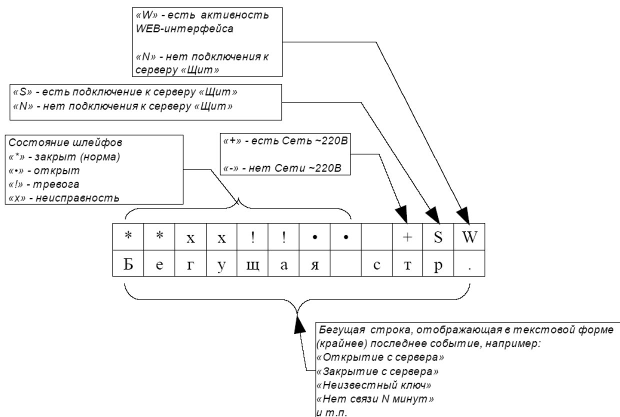
Рисунок В1 – Структура главного экрана ЖКИ
