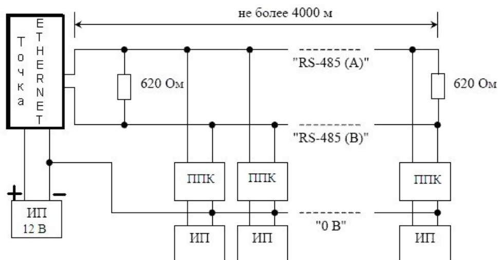
Рисунок 2 – Подключение к прибору ППКОП нижнего уровня по схеме соединения типа «шина»
